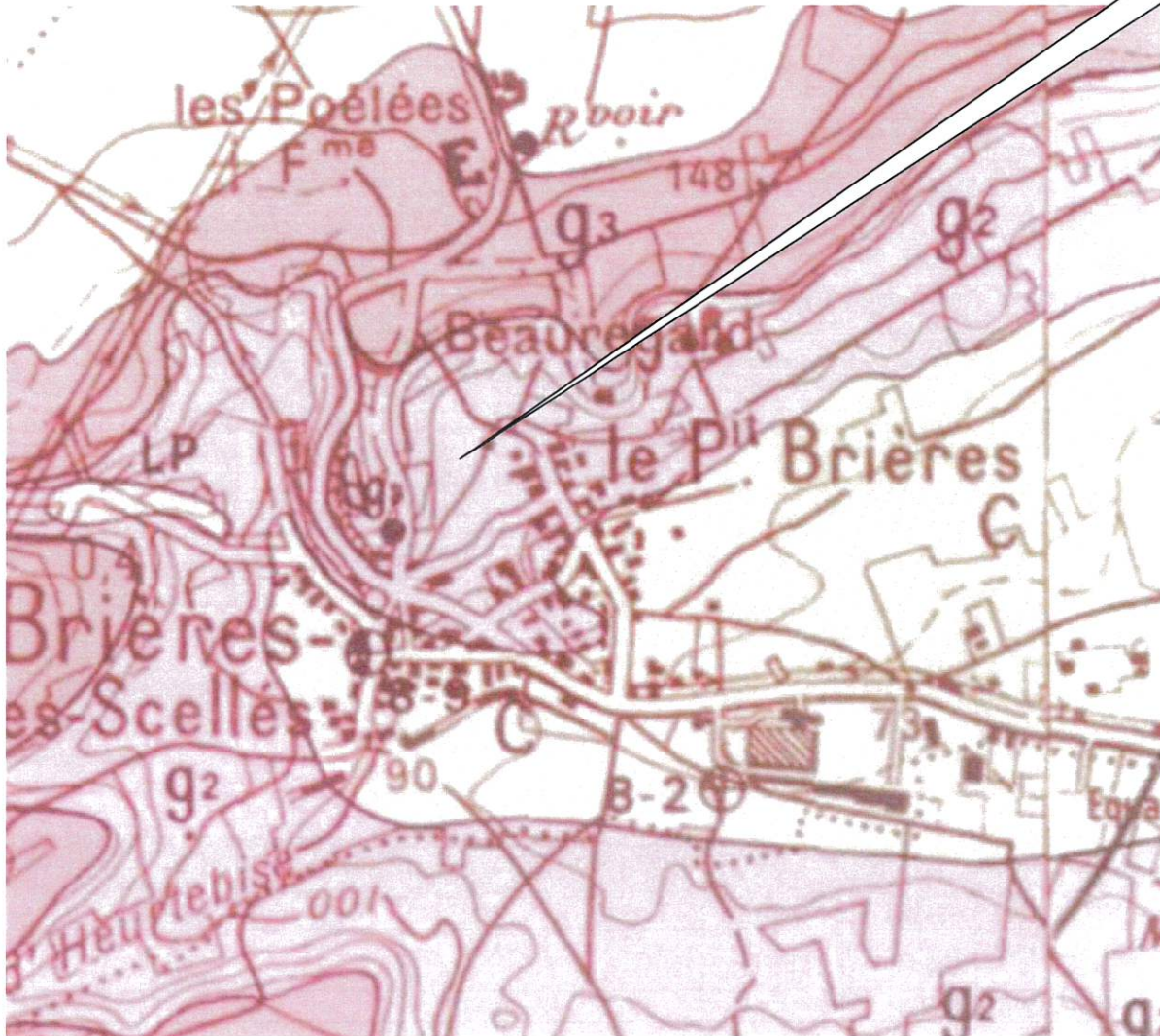
Illustration 2 : Contexte géologique général
