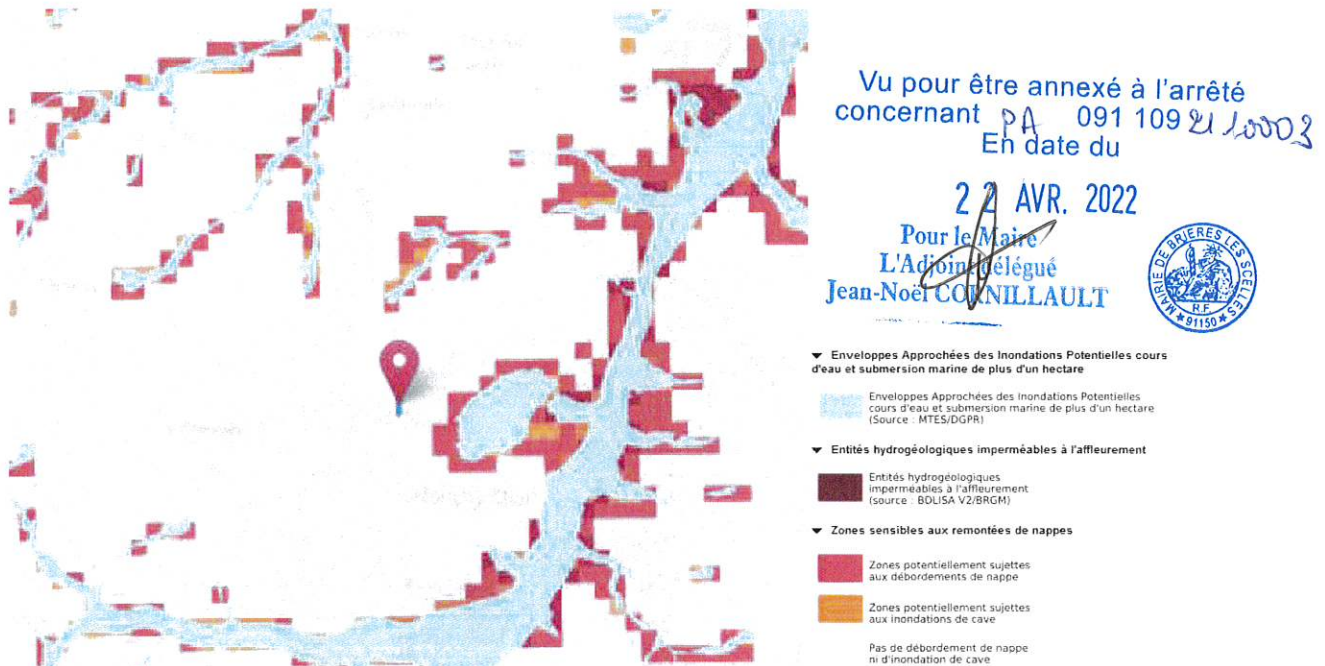
Illustration 4 : Risque de remontées de nappe
