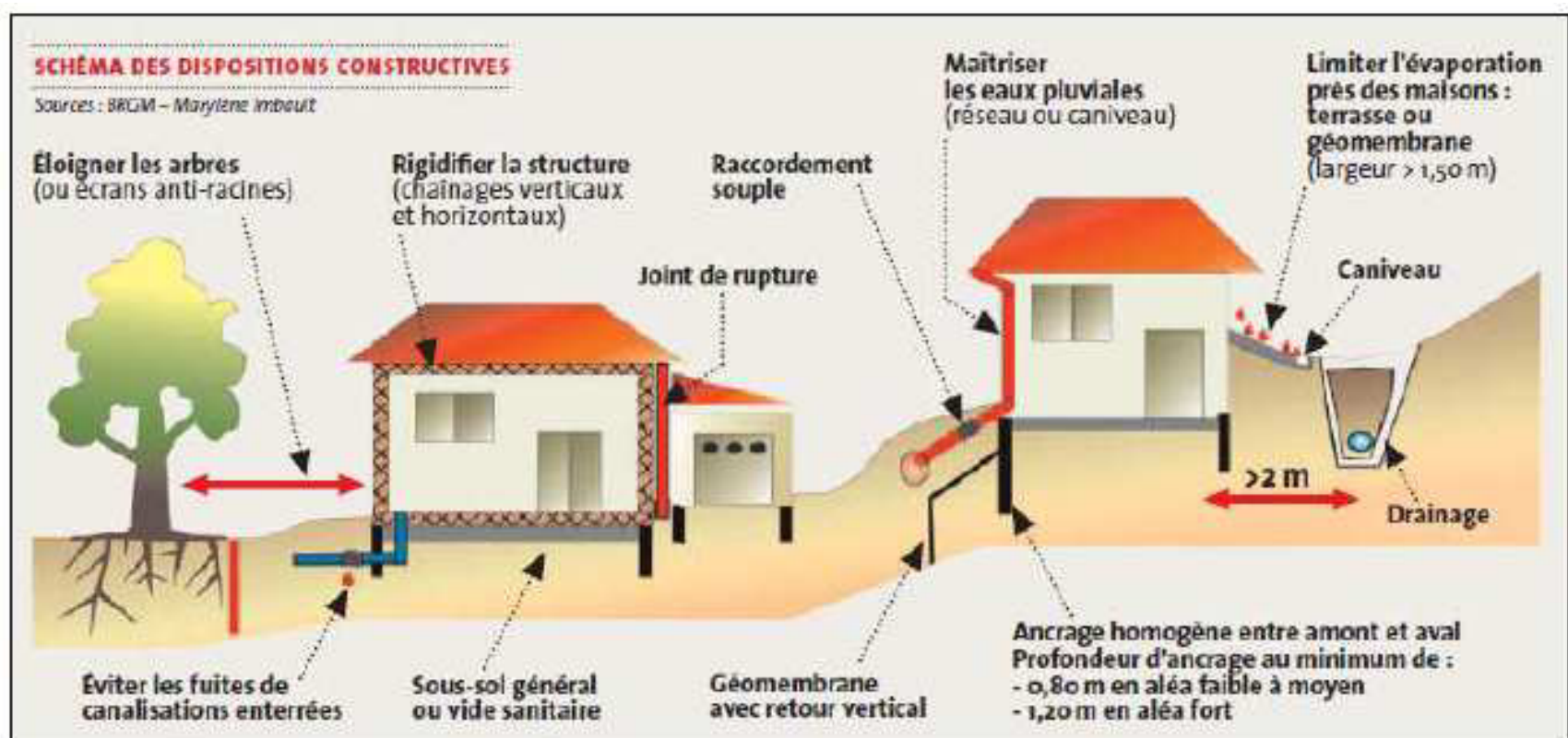
Illustration 6 : Schéma synthétique des dispositions constructives (www.georisques.gouv.fr)
