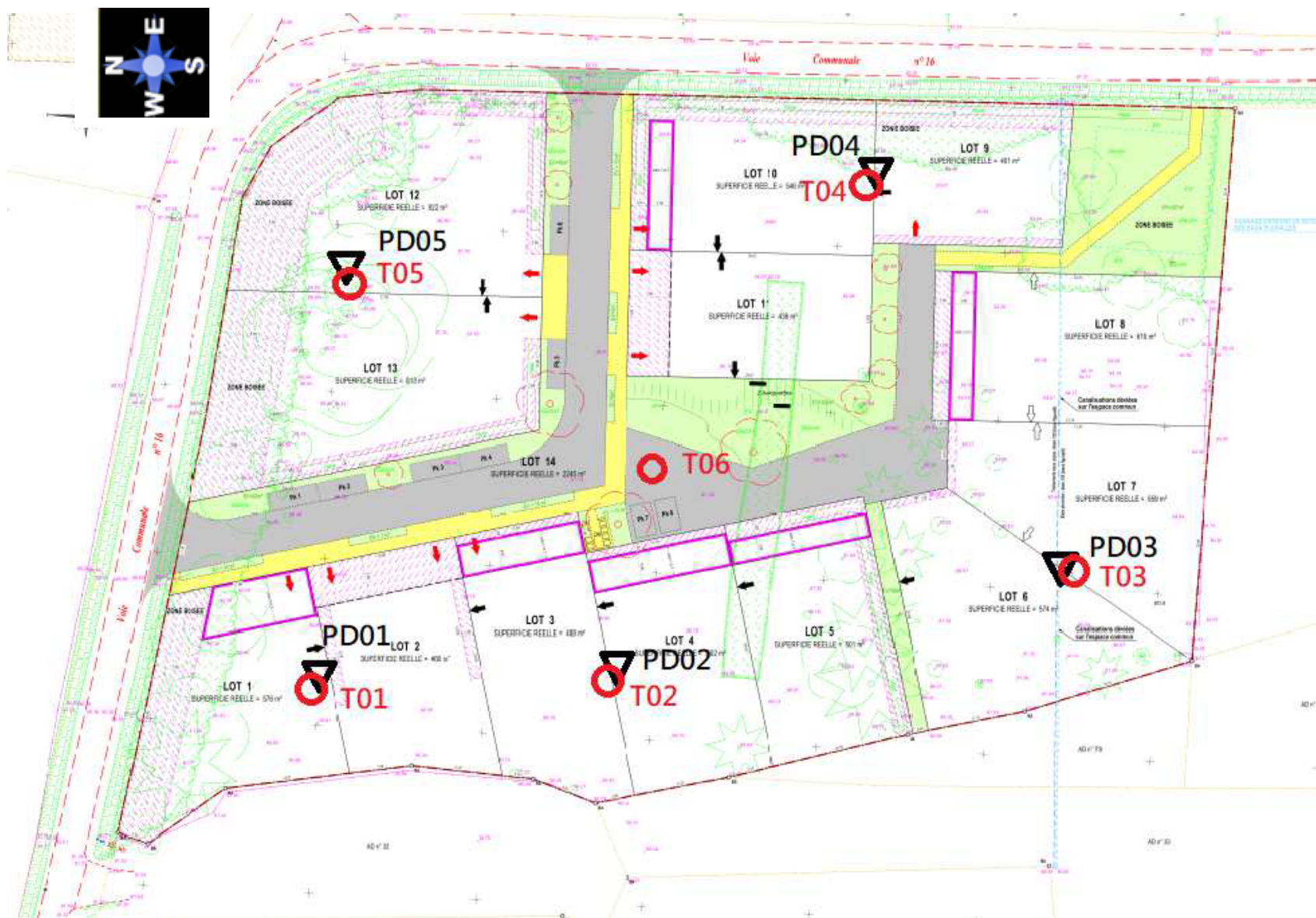
Plan 1 : Implantation des sondages
